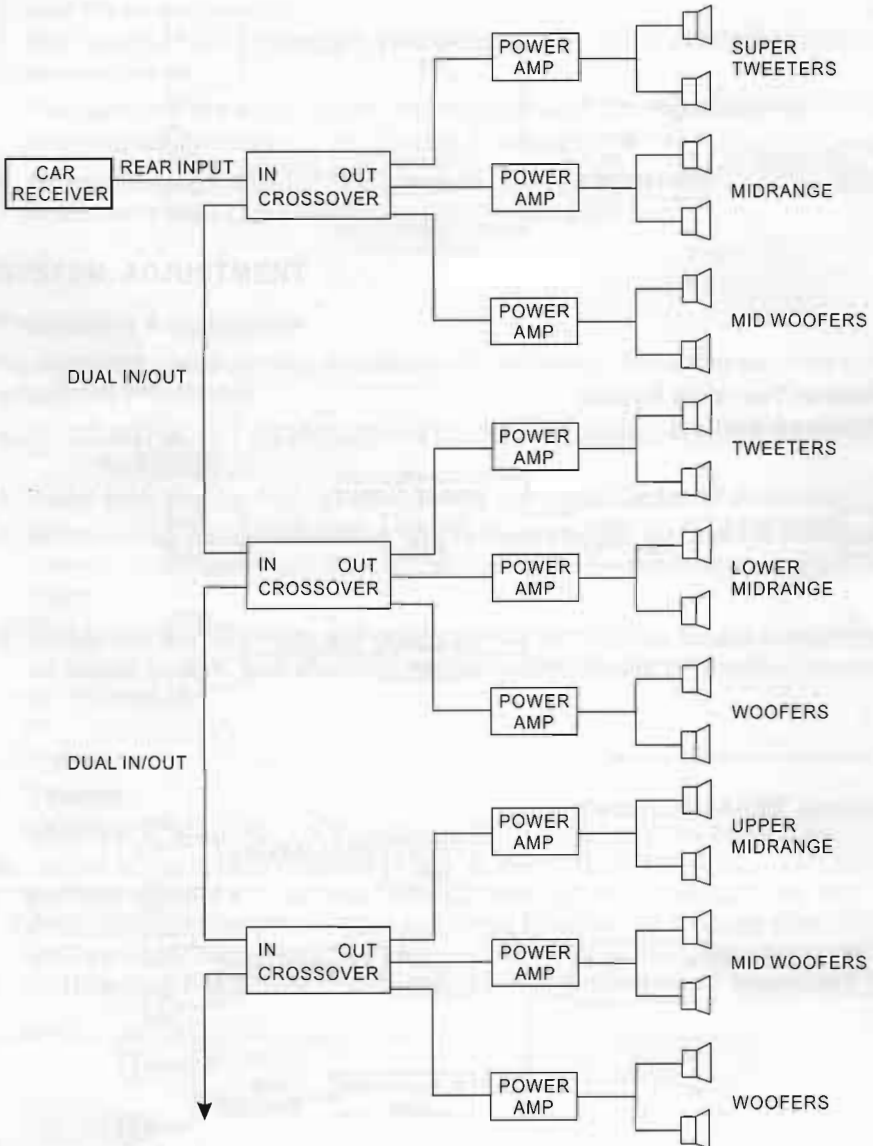
(D) 2-Channel multiple purpose system
